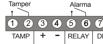
Figura 1: Bloque de terminales
